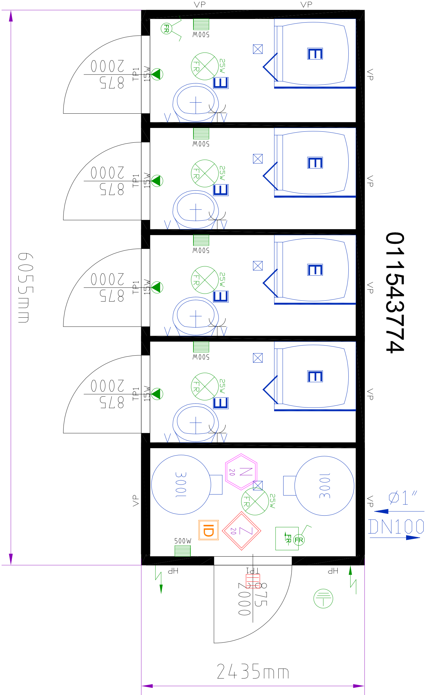
404399-004.dwg
